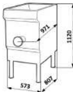
Dimensiones TX98 COMPACT
