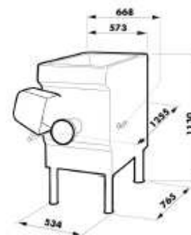
Dimensiones TX114 COMPACT
